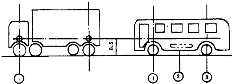
图 2 发动机噪声的测量场地和传声器位置
